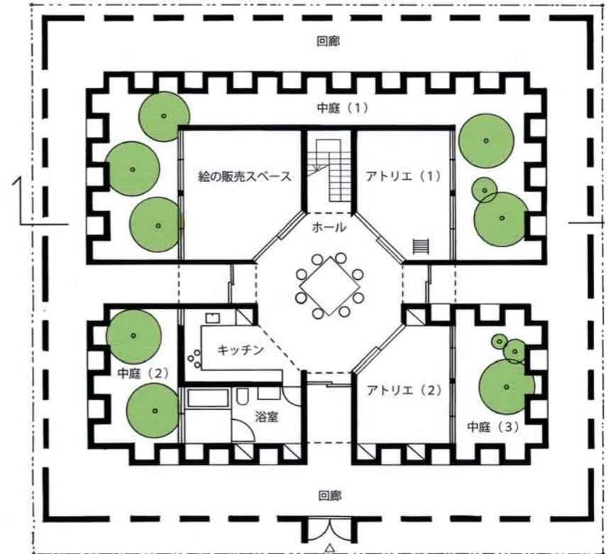
1階平面図 縮尺 1/150
